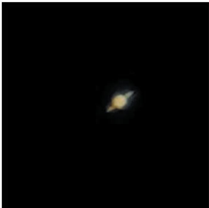
右画像：2026 年 10 月 9 日の土星
